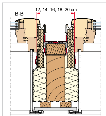
Standardní kombinace bez pomocné krokve EKS
