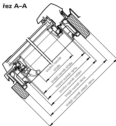
řez A-A
