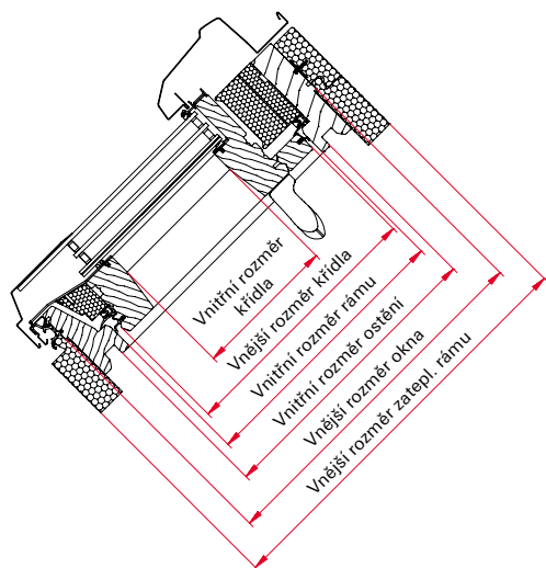
Řez A-A
