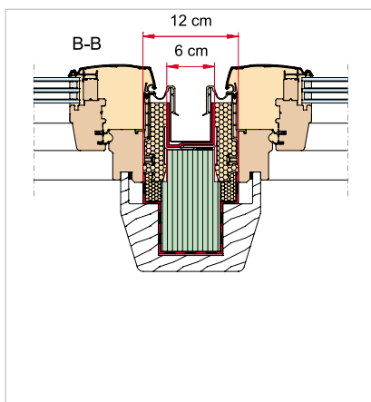
Kombinace pomocné krokve EKS s obložením z masivního dřeva v bílé barvě pro jiný systém ostění než Roto ZIN
