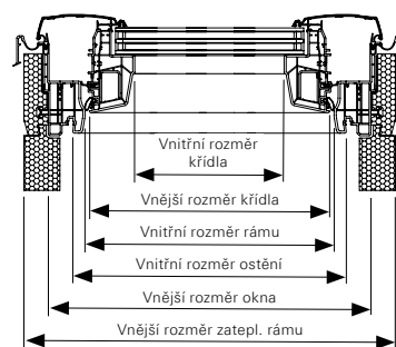
řez B-B
