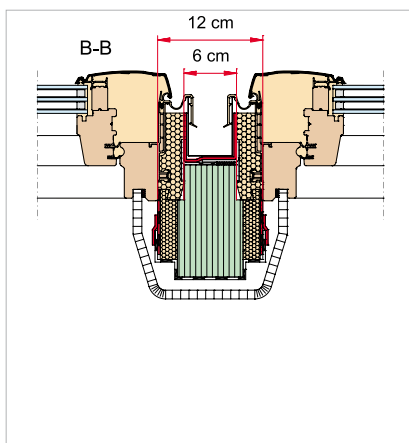
Kombinace pomocné krokve EKS s napojením na systémové ostění Roto ZIN
