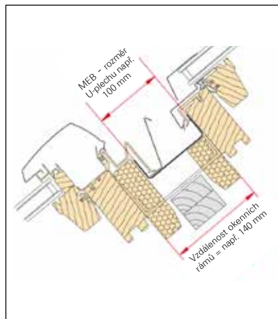
Řez oknem R4/R7
